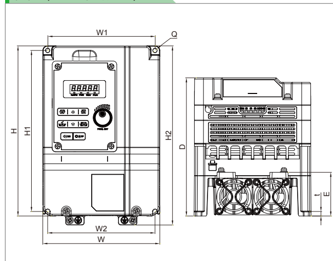
圖B (IP20框號二)
