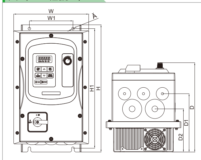
圖J (IP66框號二)
