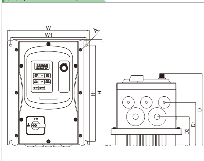
圖I (IP66框號一)
