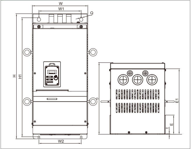
圖H (IP20框號六，含濾波器)
