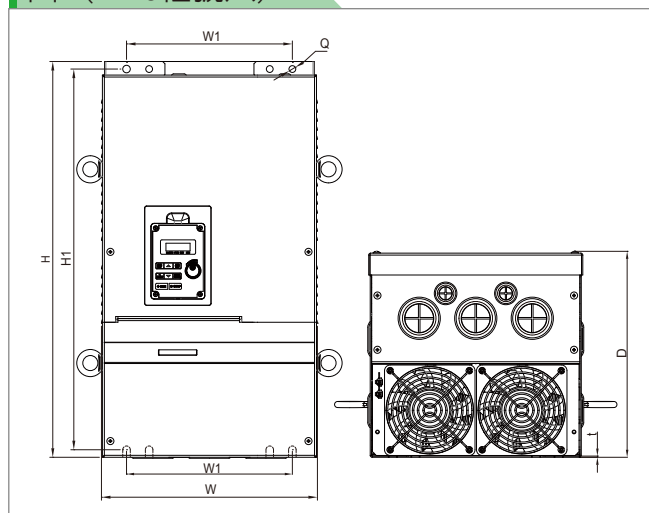
圖F (IP20框號六)
