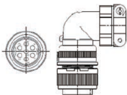
JSSCNML07 (含煞車接點) Connector MS310820-15S MS3057-12A(SR)
