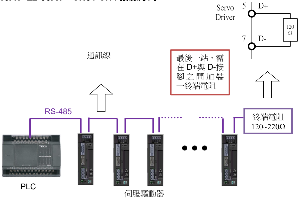
CN3 / CN4 驅動器側 PG 端子配置圖(RS-485 通訊)：
