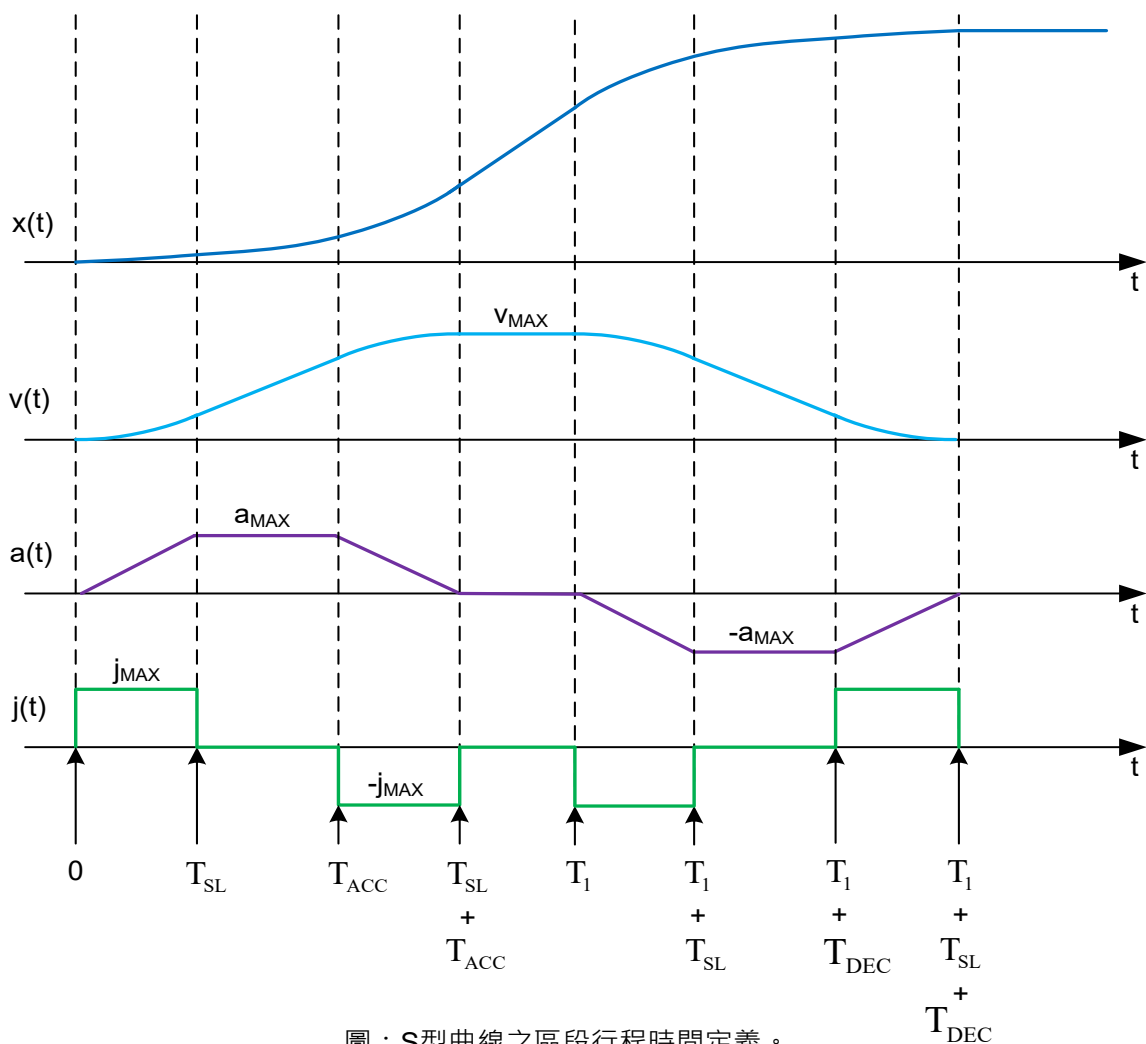
圖：S型曲線之區段行程時間定義。
